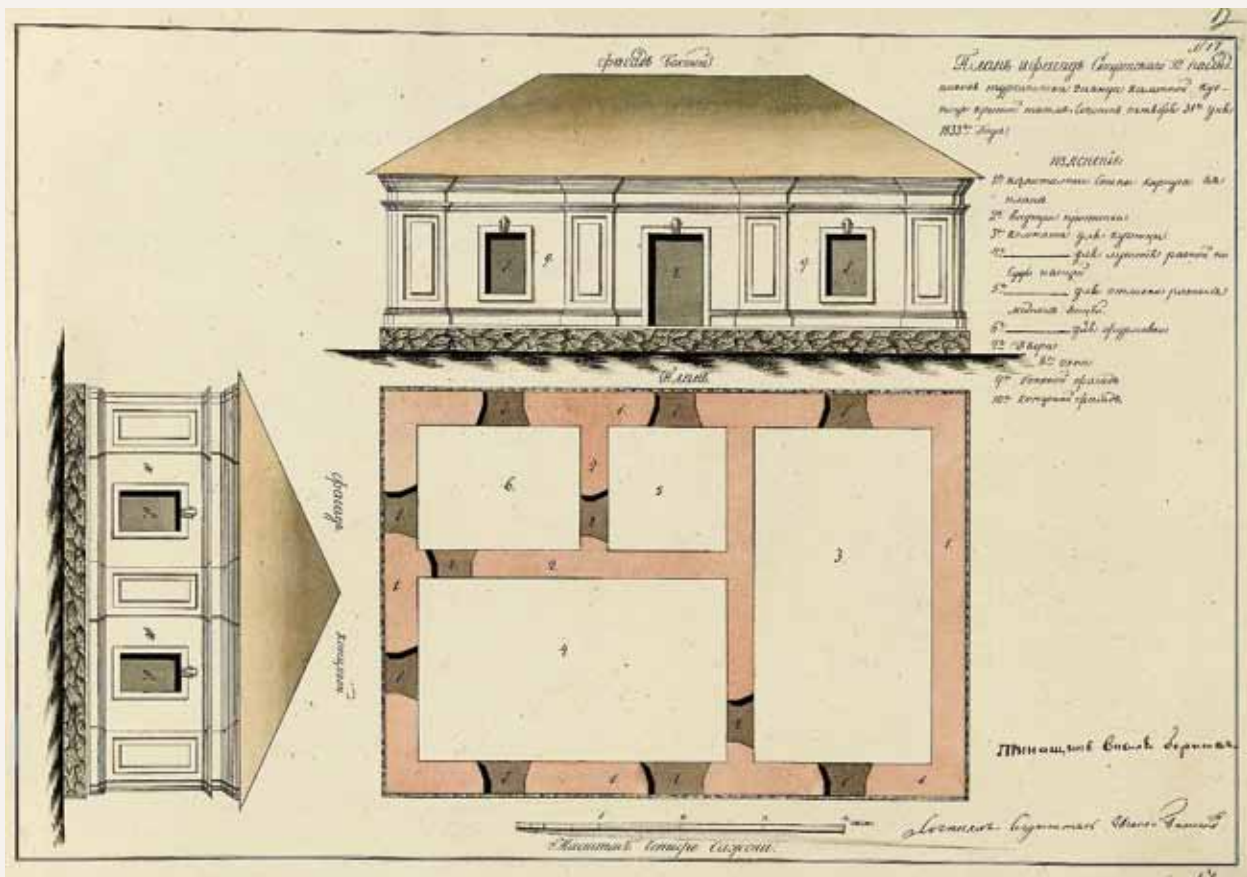
▲ Чертеж каменной кузницы, крытой тесом. РГИА Ф37. ОП63-2. Д145. Л17
